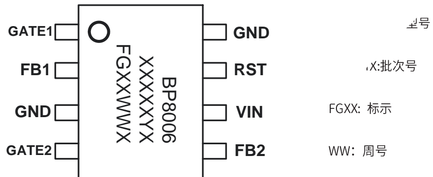
图 2 管脚封装
